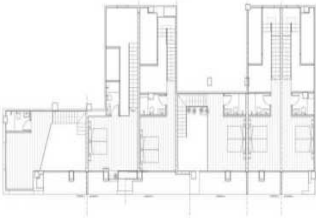
Pianta Alta
