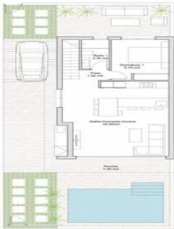
Planta baja
