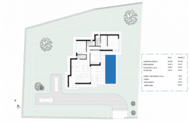
PROYECTO: MARIYLLA TITULO PLANO: SITUACION FECHA: 05-07-2021 ESCALA: 1:100 PLANO Nº: 1
