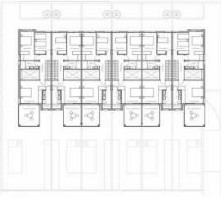
PRIMERA PLANTA
