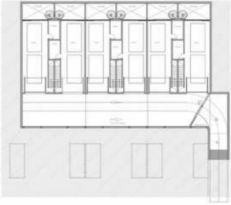
PLANTA SÓTANO
